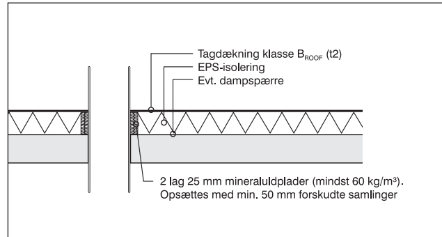
Detalje 4 - Ventilationskanal eller tagbrønd
