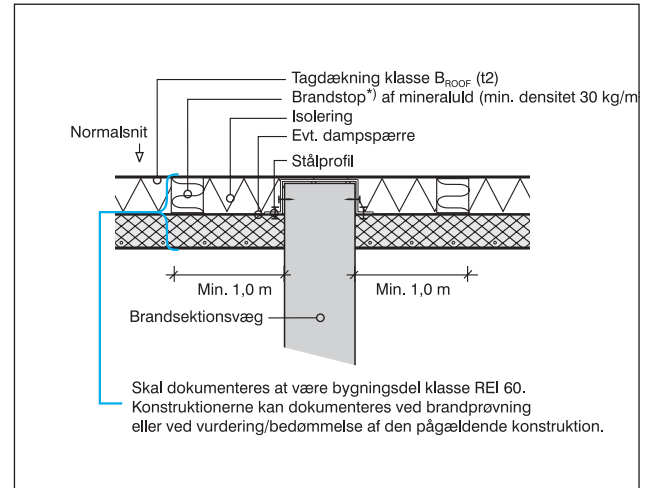
3.2 Brandkammerstatning
