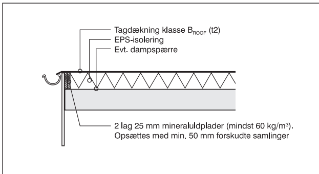
Detalje 1 - Stern
