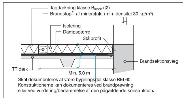
2.4 Spring i bygningshøjde
