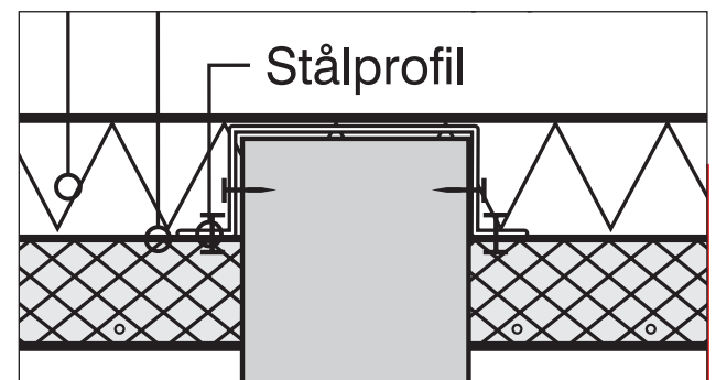
3.2 Brandkammerstatning FORSTØRRET
