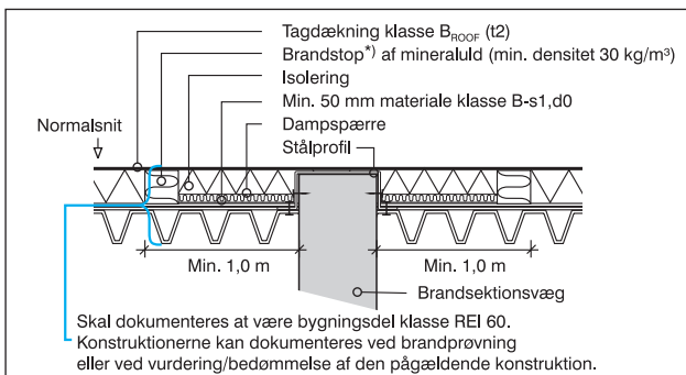
1.3 Brandkammerstatning
