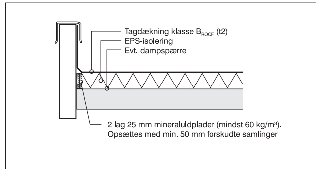
Detalje 2 - Stern
