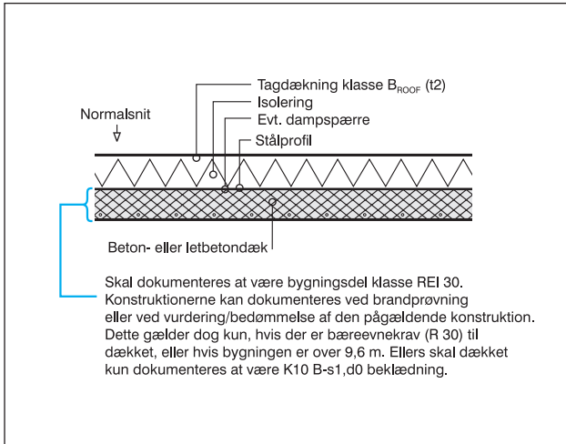
3.1 Normalsnit
